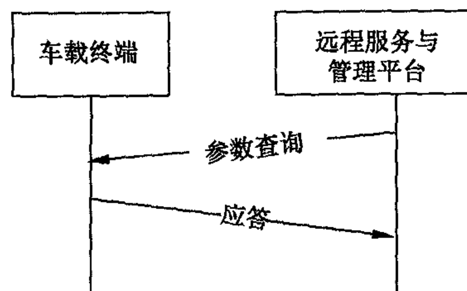
图 B.4 参数设置流程示意图
