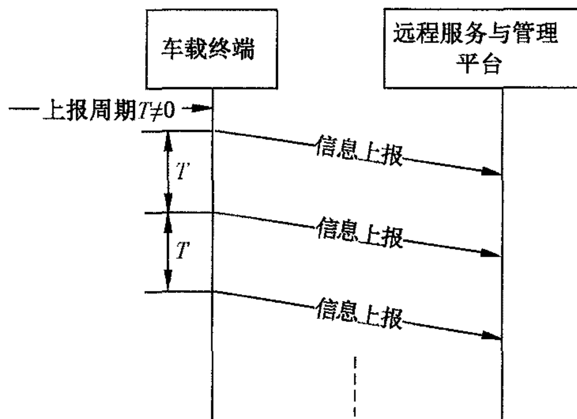
图 B.2 实时信息上报流程示意图
